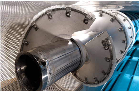
Snekketransportør i perforeret stålkar.
