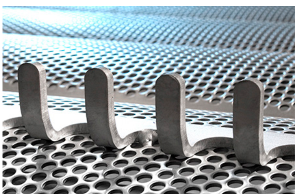
Elementer til transportbånd fremstillet af kantbukkede og valsede perforerede plader.
