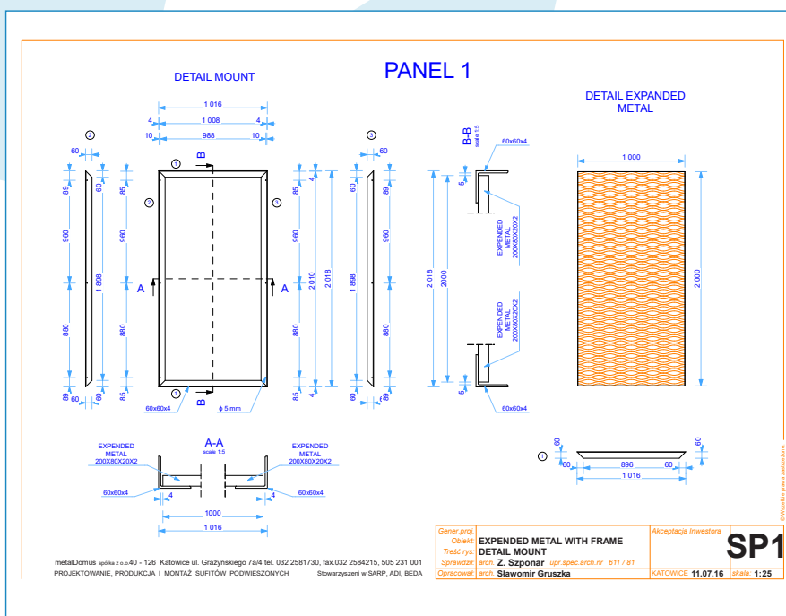
Eksempel på produktionstegninger.
