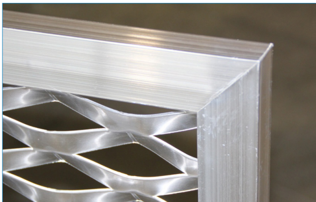
Strækmetal svejst i vinkelramme.
